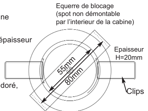
DÉCOUPE 55MM DIAMÈTRE EXT 80MM
