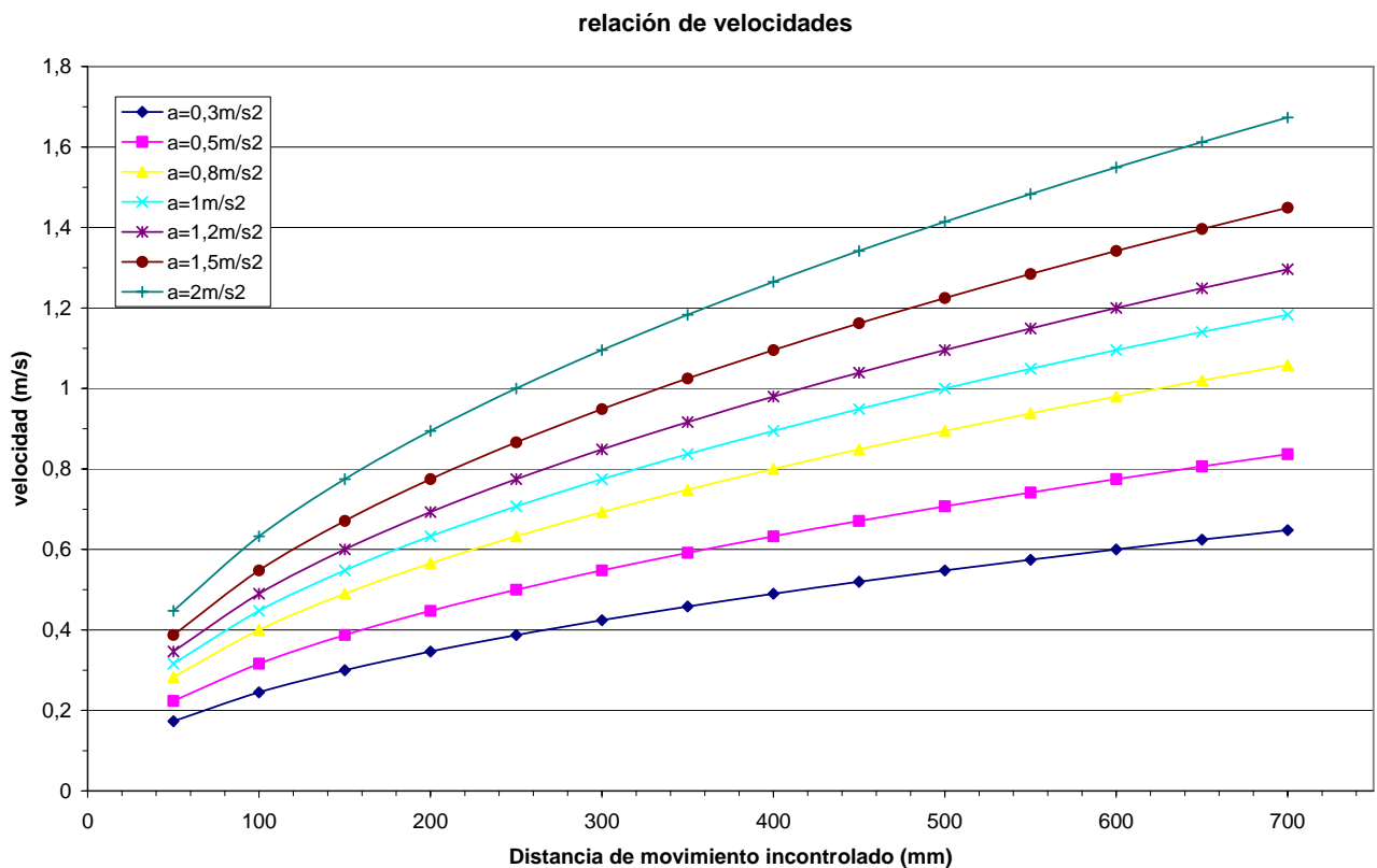
Img 1. Graphique de rapport de vitesses
