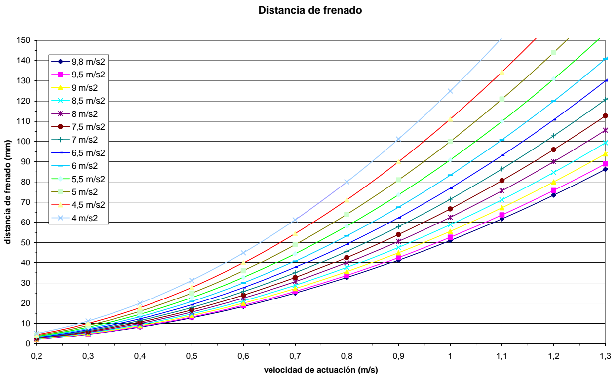
lmg 2. Graphique pour obtenir la distance de freinage des parachutes
